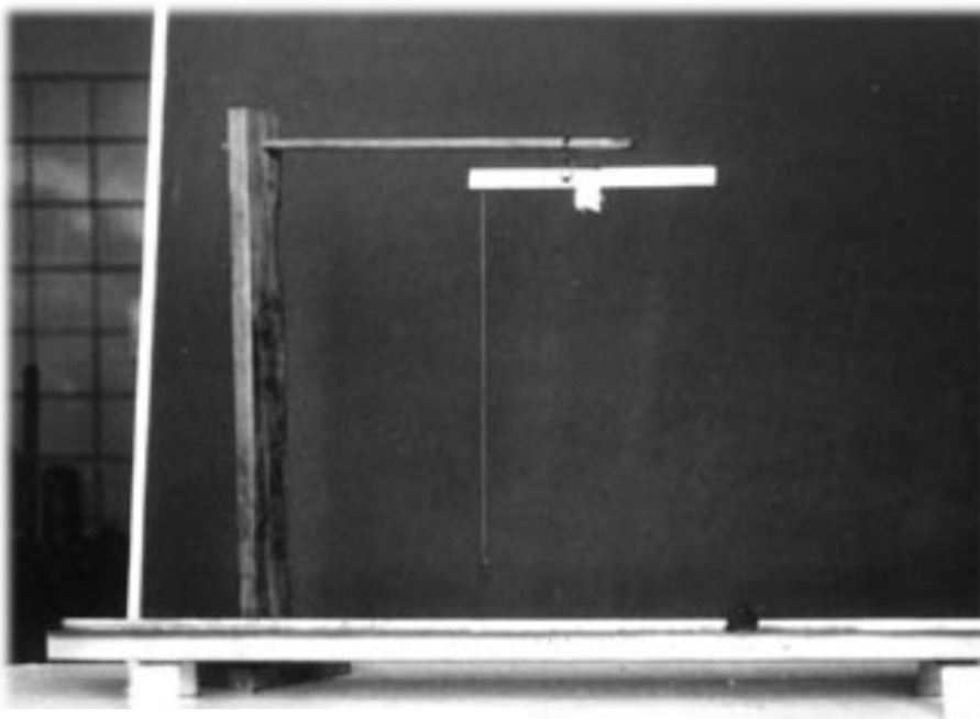
Nachbau einer Schieberrinne.
